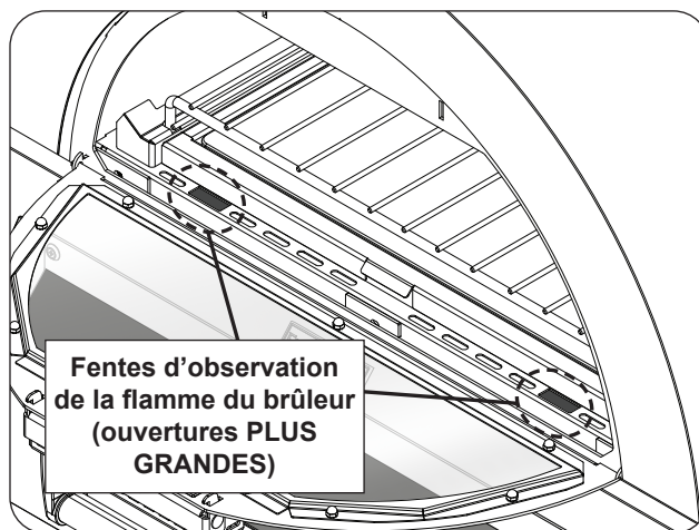
Fig. 34-3 Orifices d'observation de la flamme du brûleur
