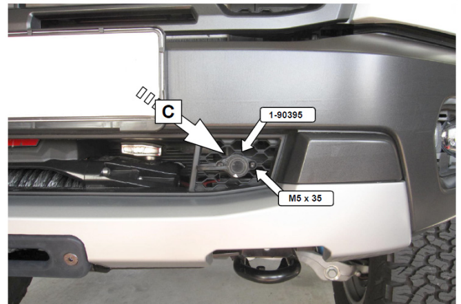
26 Steckdose einsetzen! / Mount the socket! Teil „C“ hinter dem Gitter / Part „C“ behind the grid
