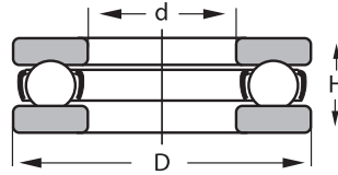
Enkelverkande
