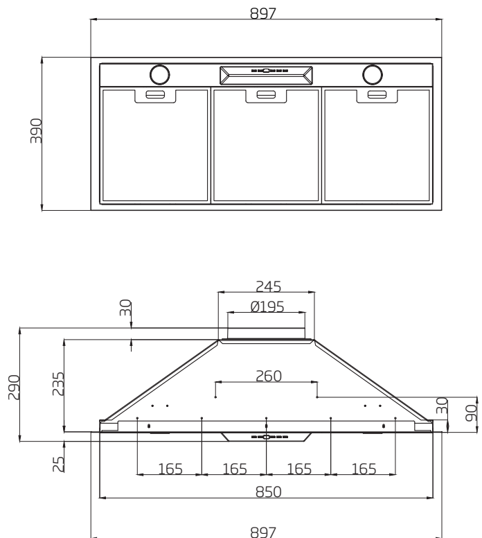
UM1390-9BS // 90cm AIR OUTLET ø200
