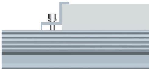
Endklammer
