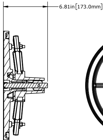
SECTION A-A SCALE 1 : 6
