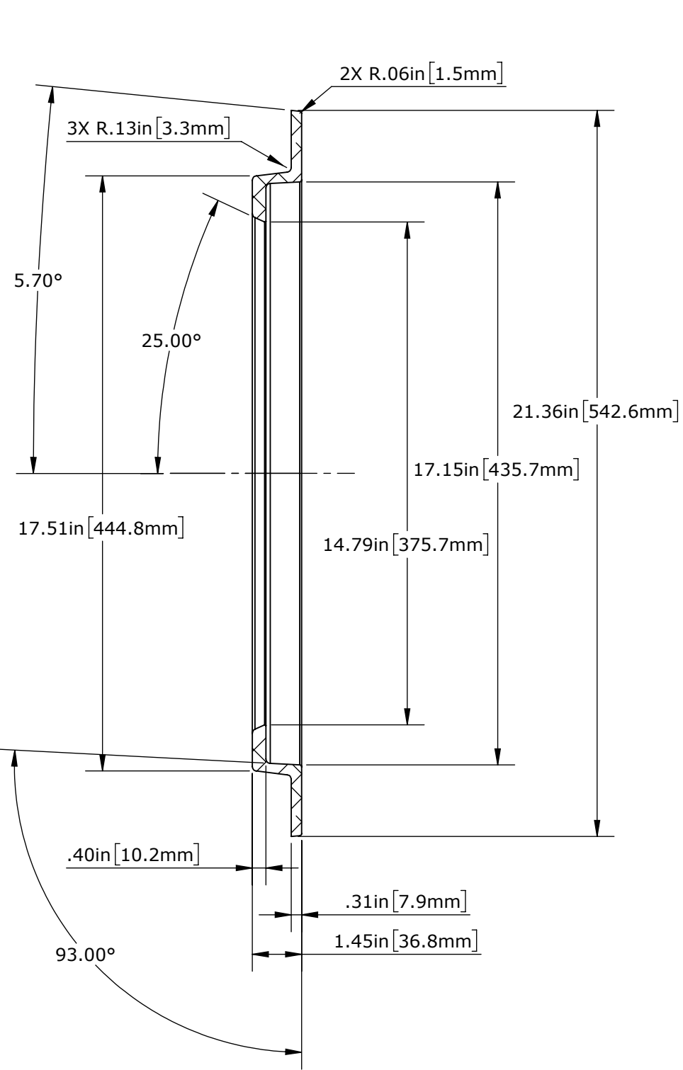
SECTION A-A
