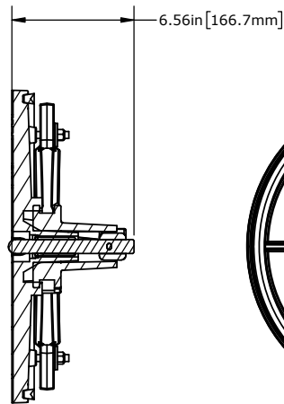
SECTION B-B SCALE 1 : 6
