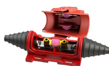
Mini ANL fuse mounting
