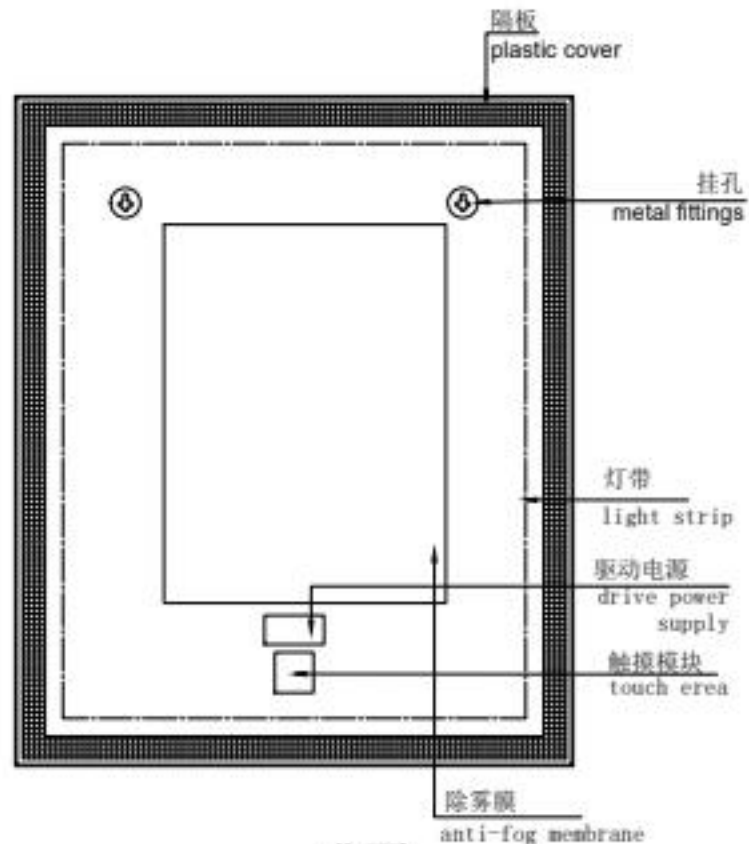
背面 backside
