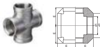
Keturšakis 10 bar
