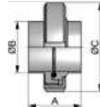
Trumpa versija
