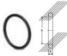
O-žiedas
