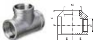
Trišakis 10 bar
