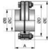
Trumpa versija
