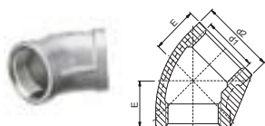
Alkūnė 45° 10 bar
