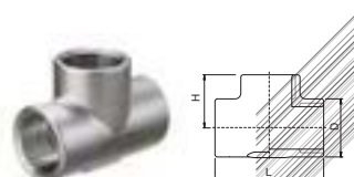
Trišakis 40-100 bar
