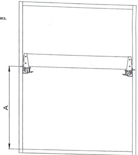
ES. Cassetto Blum tandembox. E.G. Blum tandembox drawer.
