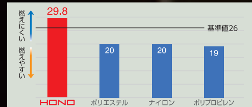
素材別燃焼指数 (LOI値)
