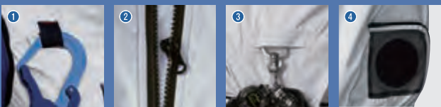
1 2 掛付け対応フック掛け 2 引っ張るだけで外れるクイックフリーファスナー 3 ランヤード取り出し口 4 ファン落下防止ネット付(ファスナー付)
