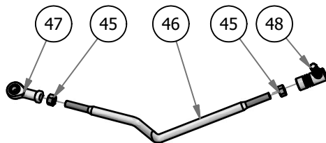
035-5451-00 Push Rod-Left
