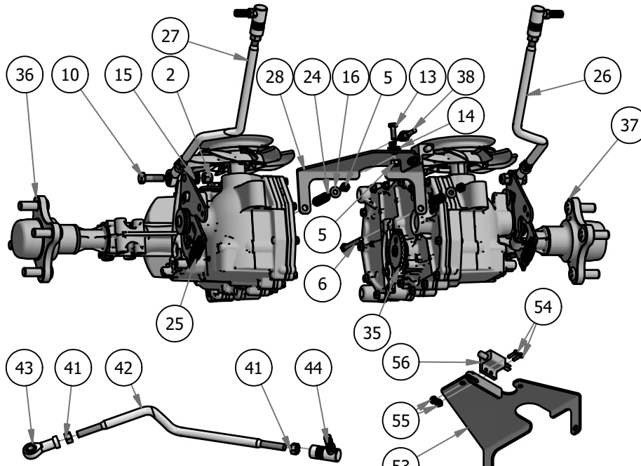
035-5450-00 Push Rod-Right
