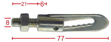
ANTI-LOOSE FASTENER MINI BOLT ON SH-171 Zinc
