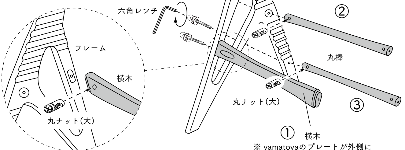
横木取り付け方法
