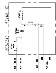
6E MOTOR SCHEMATIC FIG. 4
