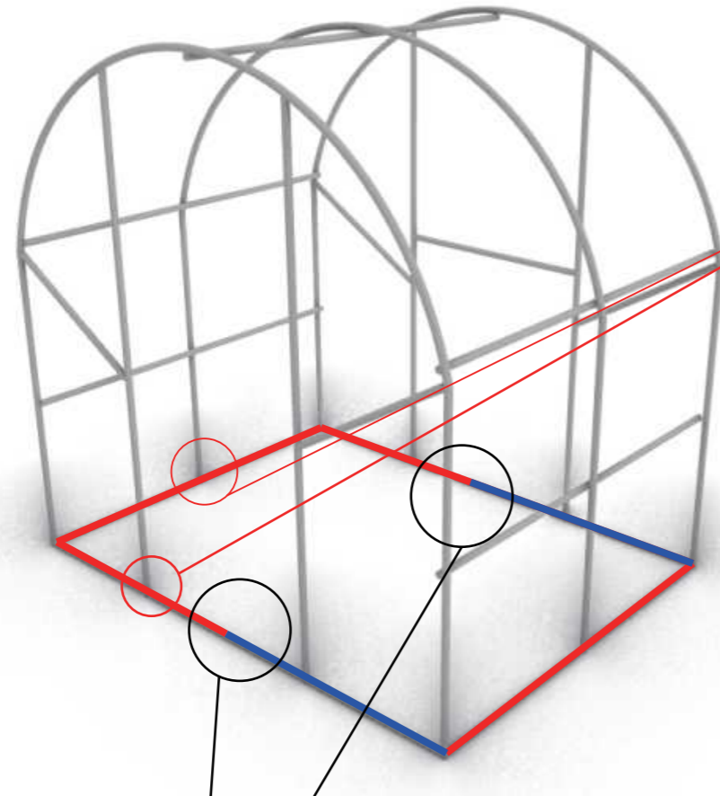
21、 Self Screw
