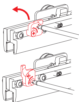
Activation anti-release Attivazione antiganciamento
