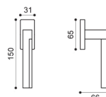
MP 15/R Maniglia per finestra D.K. Window handle D.K.
