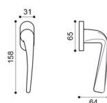
LM 15 Maniglia per finestra D.K. Window handle D.K.
