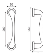
LM 20 Maniglione. Pull handle.
