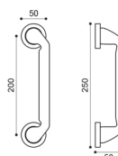
DY 20 Maniglione. Pull handle.
