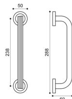
CD 20 Maniglione. Pull handle.
