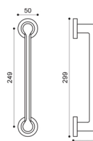
AR 20 Maniglione. Pull handle.
