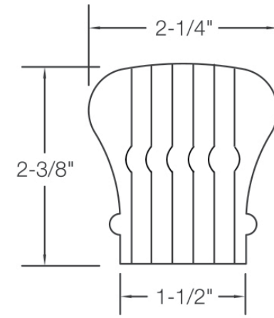
6010B Profile
