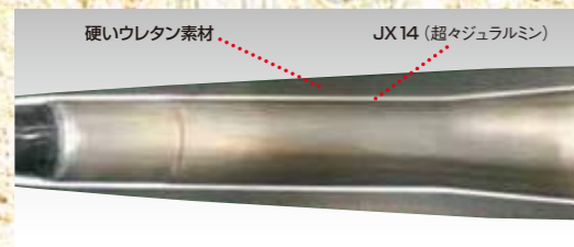
ハーフ&ハーフ断面図:3層構造
