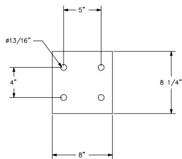
DETAIL A-A (TYP)
