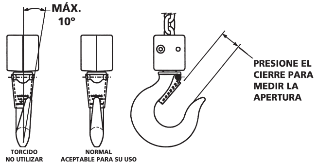
Figura 3 – Inspección del gancho
