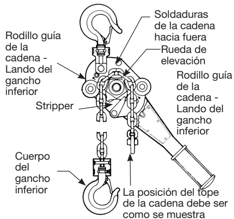
Figura 11 - 3/4, 1, 1 1/2 y 3 Tonelada
