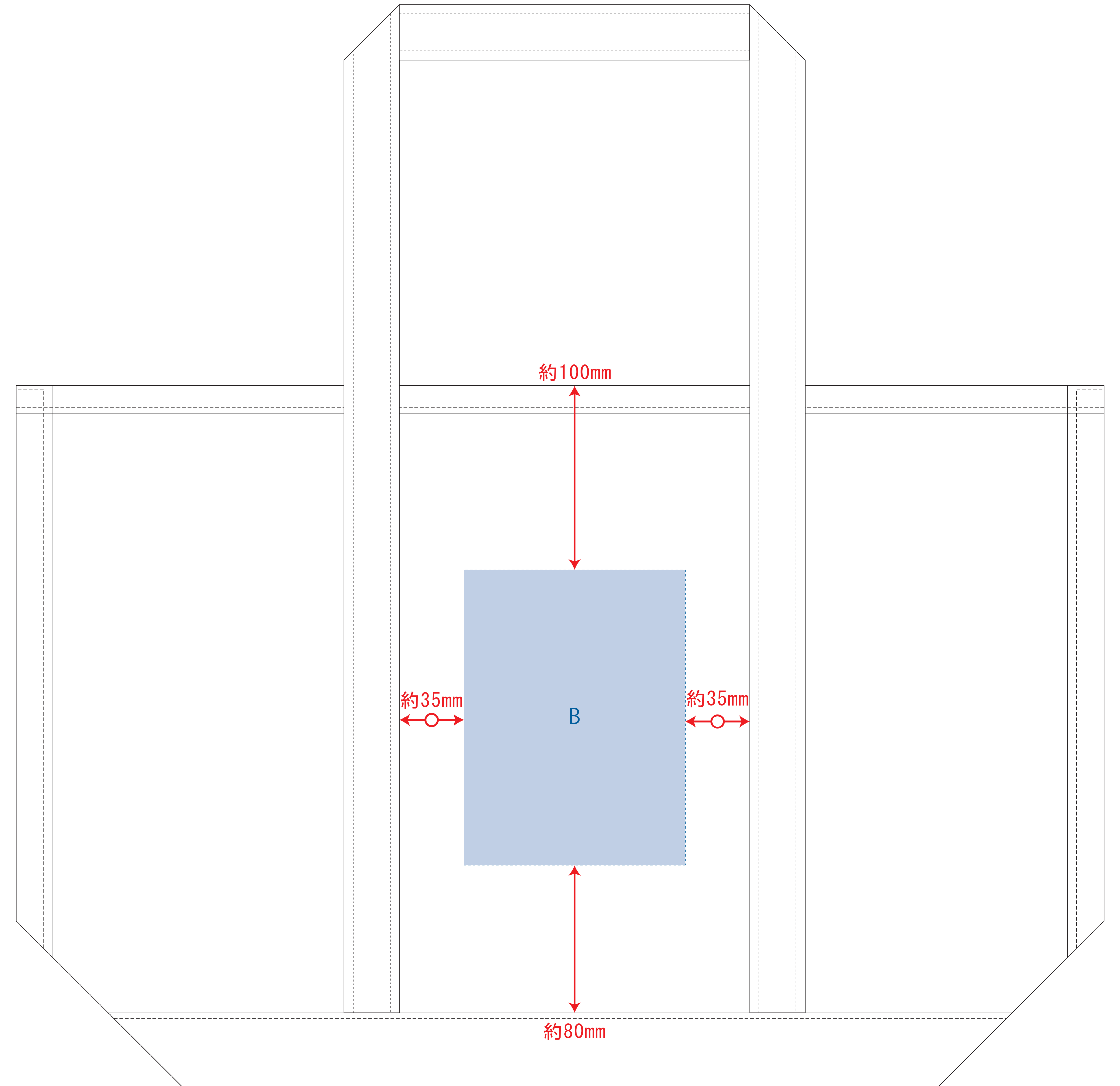
背面
