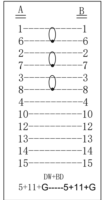
接线图:
