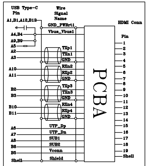
WIRING TABLE
