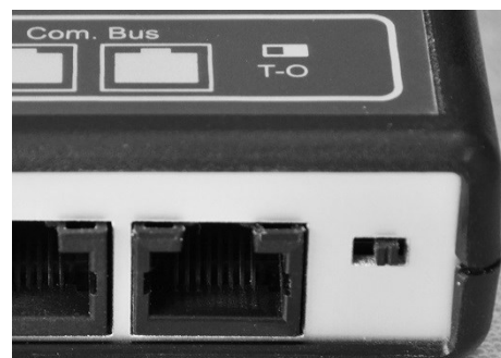
Terminaison BSP désactivée (position O)
