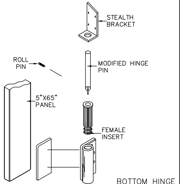
BOTTOM HINGE
