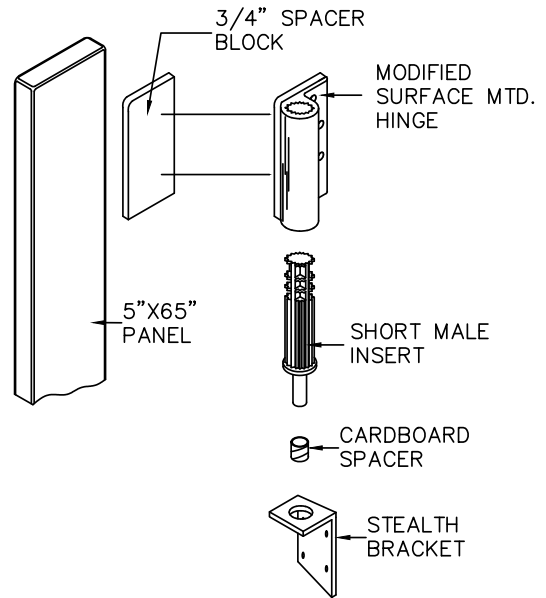
TOP HINGE
