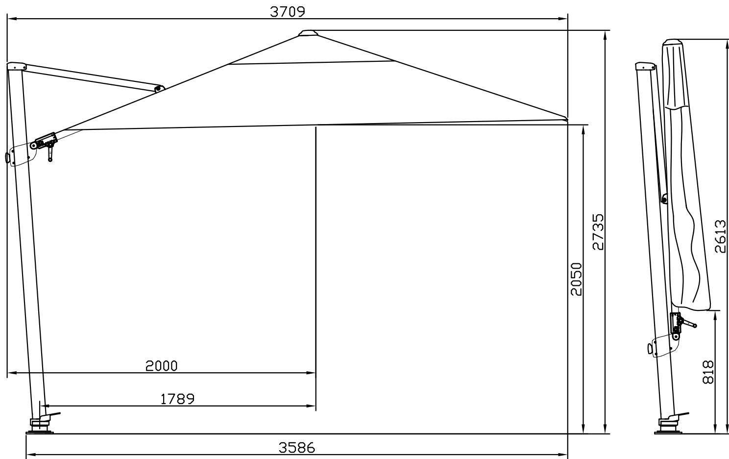
AG25R-35伞形图 配C-42-190
