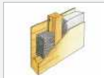
Hohlraumverfüllung und Dämmung im Holzrahmenbau
