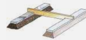
Liaporfitstreifen mit Waaglatte: in den Zwischenraum eingefülltes Liaporfit mit Waaglatte abziehen.
