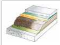
Belastbare Schüttung auf Massivdecke mit Nass-Estrich* als obere Abschluss
