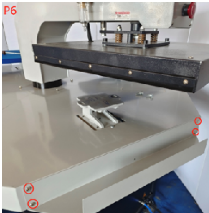
P6 : Installez le bac à tissu (il est conçu pour les longs travaux de presse à tissu, ce qui peut empêcher le tissu de tomber, cette pièce pourrait ne pas être nécessaire pour une presse à t-shirt régulière)
