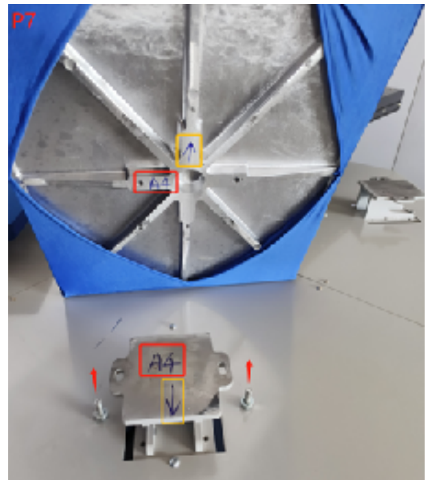
P7 : installez le plateau, faites correspondre la marque (A4-A4) et la direction. Nous avons pré-aligné le plateau pour le rendre parallèle à la plaque chauffante afin d'assurer la meilleure répartition de la pression. Fixez le plateau avec une vis, une rondelle élastique et une rondelle plate.
