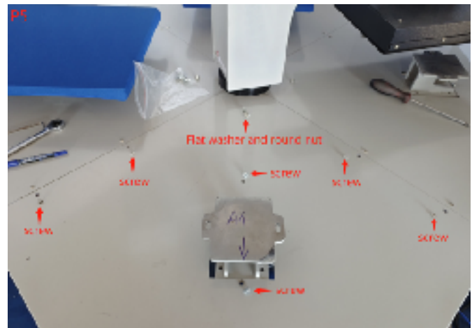
P5 : Fixez les quatre couvercles avec des vis comme indiqué sur l'image.
