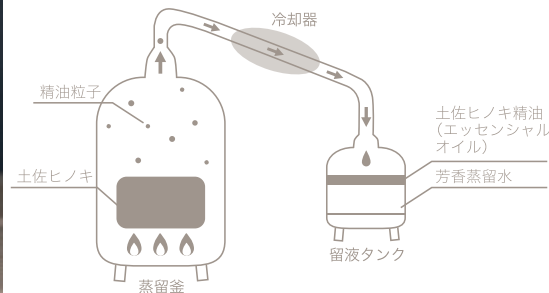
※水蒸気蒸留のイメージ
