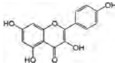
Kaempferol
