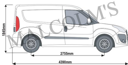
Fiat Doblo 2010-2021 L1H1.jpeg
