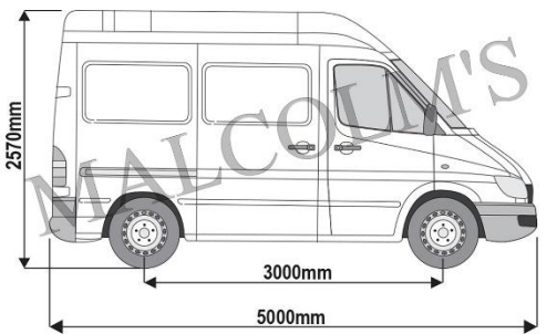
Mercedes Sprinter 2000-2006 L1H2.jpeg
