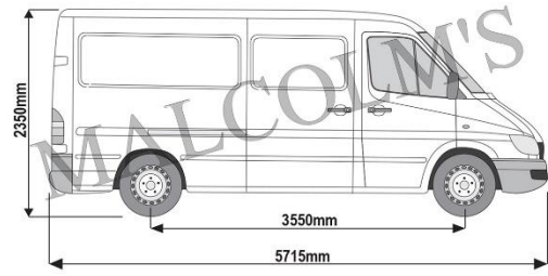
Mercedes Sprinter 2000-2006 L2H1.jpeg
