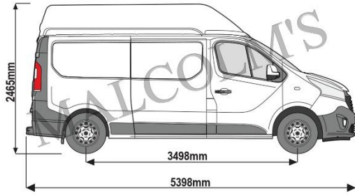
Nissan NV300 2016-2021 L2H2.jpeg
