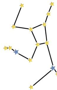
Hercules
