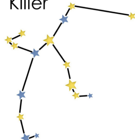
Perseus
