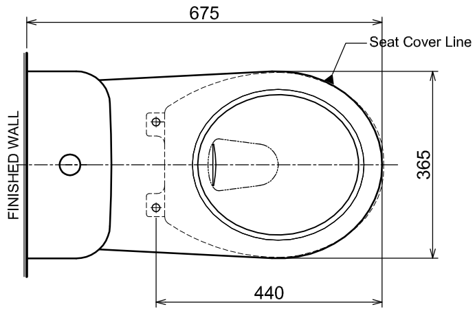
TOP ELEVATION
