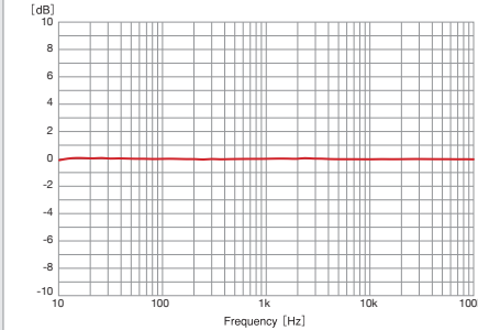
RIAA deviation (MM input)
