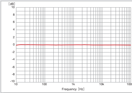
RIAA deviation (MC input)
