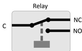
Relais-Konfiguration
