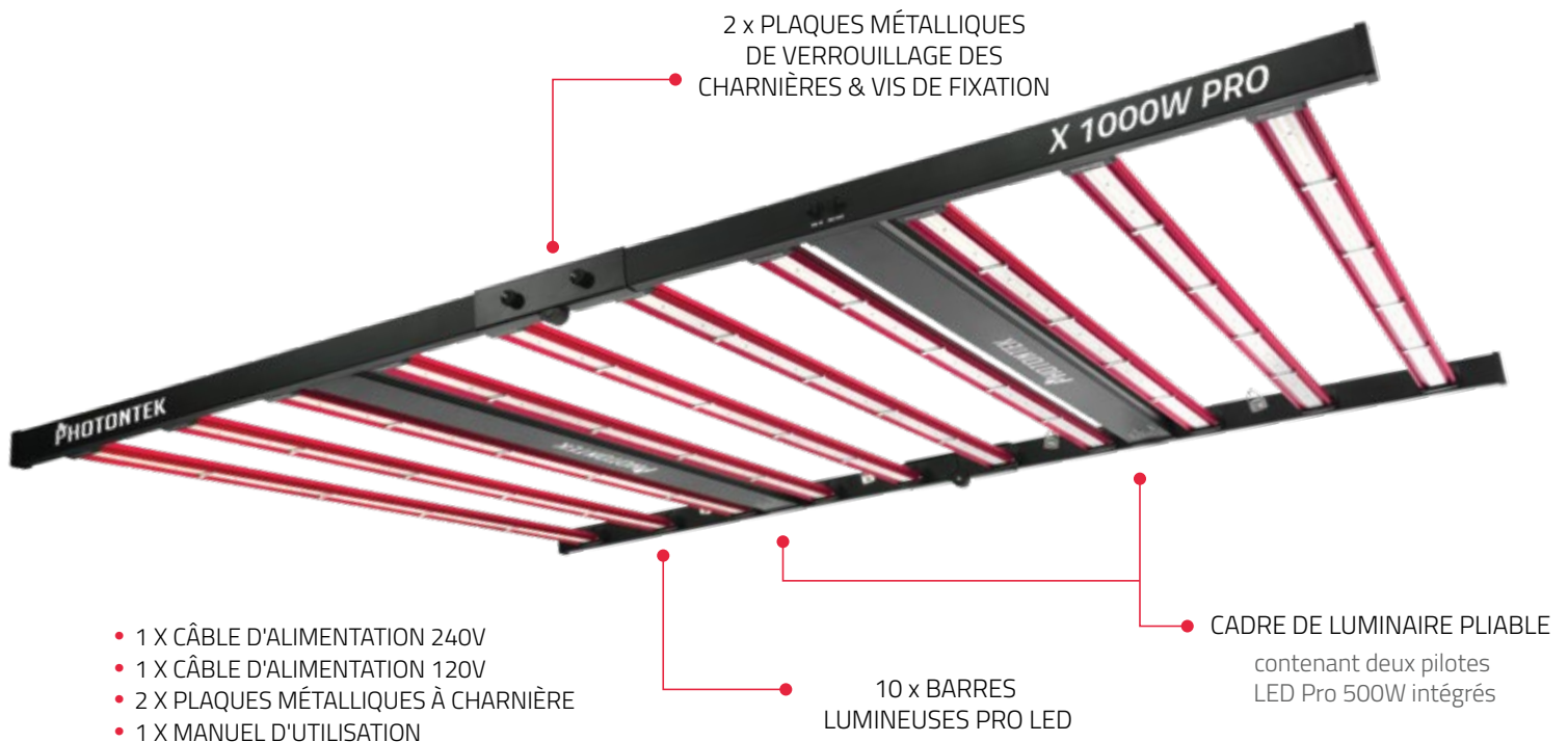
Fig4. Composants de la lampe.
