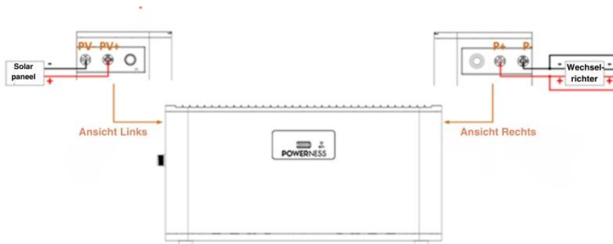
Abbildung 3-8 M01 Batterie-Schaltplan
