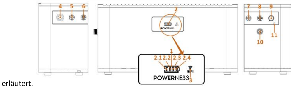
Abbildung 2-1: Geräteschnittstellen der Front- Seitenplattenschnittstelle
