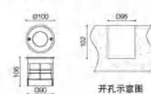
开孔示意图
