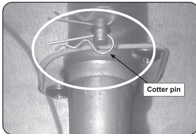
Fig. 51-1 Remove cotter pin
