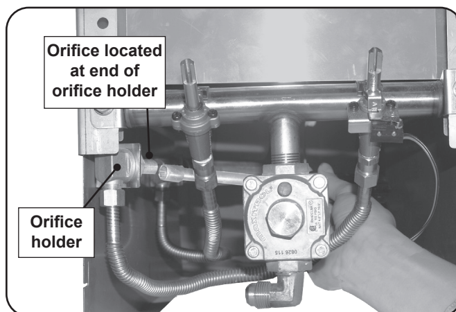
Fig. 51-3 Locate orifice
