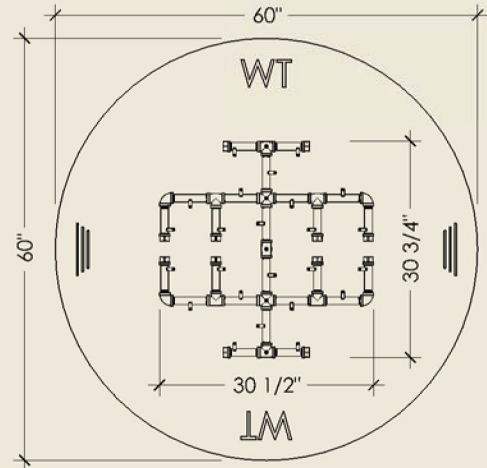
TOP ELEVATION
